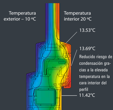
Corona AS 60 Termografía de la sección
